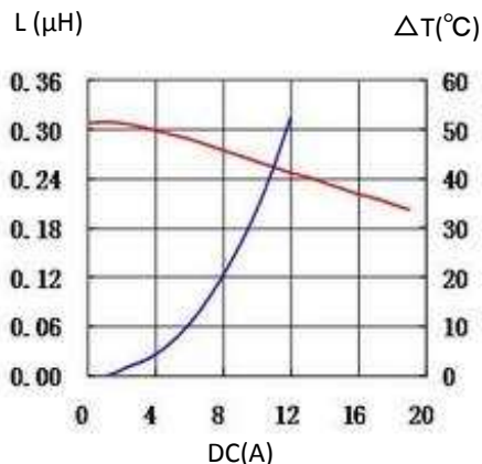
3. 0512CDMCCDS-R33MC
