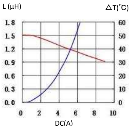
8. 0512CDMCCDS-1R5MC
