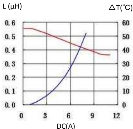
5. 0512CDMCCDS-R56MC
