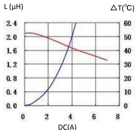
9. 0512CDMCCDS-2R2MC
