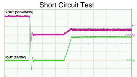
Time-200μs/div
