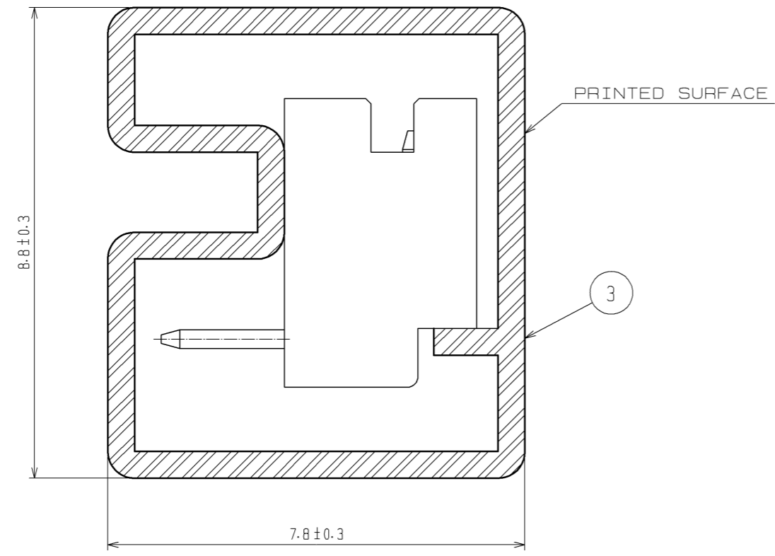
A-A (10:1)
